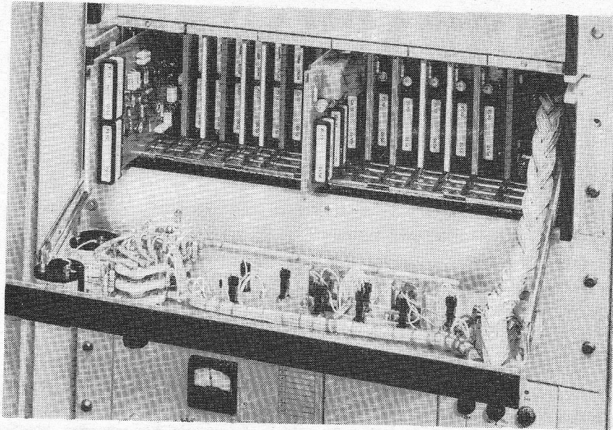
Afb. 2. De servoversterkers, gemonteerd op kaarten met gedrukte bedrading in een 19-inch standaardrek.
