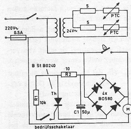
Fig. 3. Schakeling van het lasapparaat.
