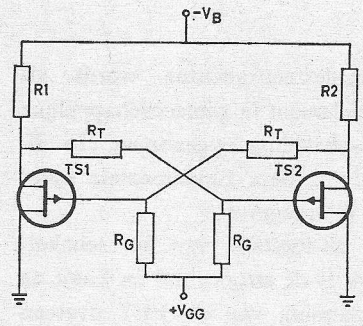
Fig. 3. Flipflop
