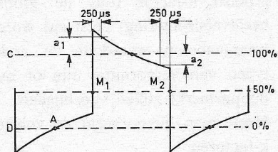
Fig. 25. Bepaling van de k_{50Hz} -factor
