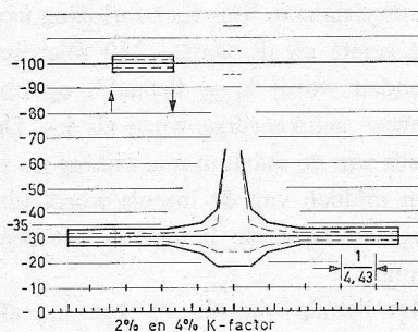
Fig. 26. Voorbeeld van een bestaand sjabloon (TEKTRONIX) voor het meten van de \sin^2 -impuls
