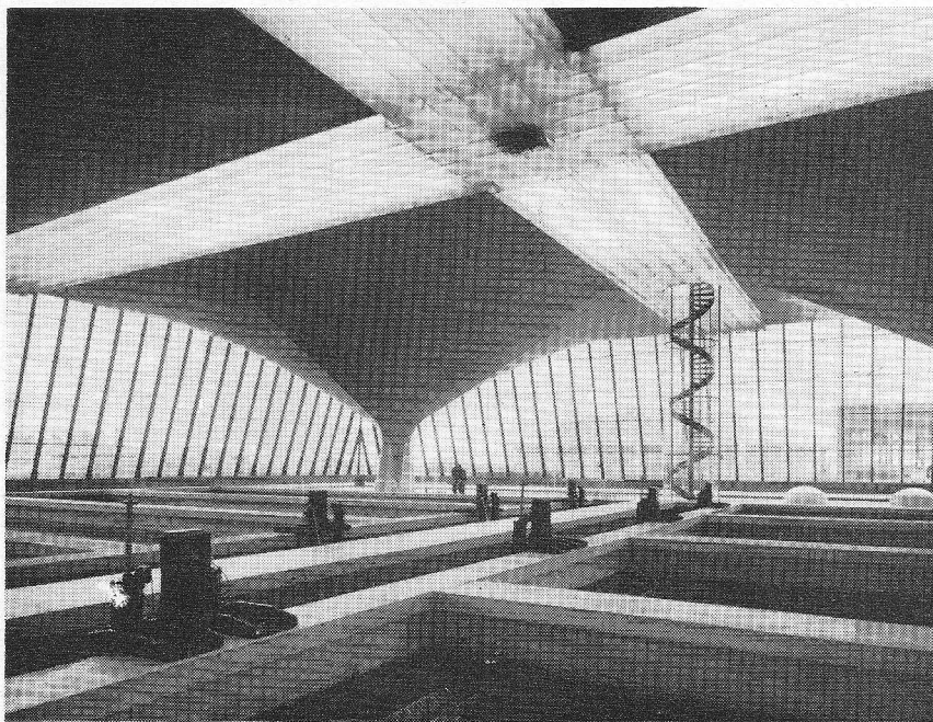
Afb. 4. Detailopname van het filtergebouw met snel- en vlokkenfilters. Op de achtergrond een deel van het machinegebouw.
