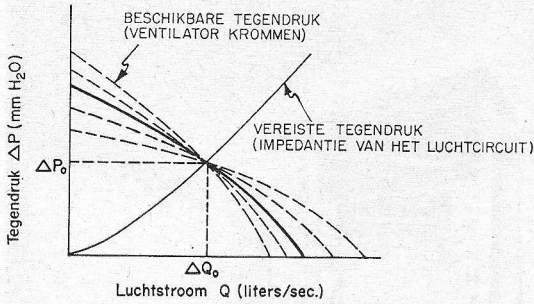
Fig. 2. Ventilator levert luchtstroom \Delta Q_0 in systeem waarbij vereiste tegendruk gelijk is aan beschikbare tegendruk = \Delta P_0
