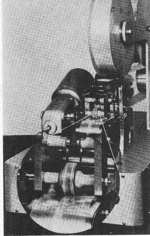
Afb. 2. Model van een kunststoffolie lasapparaat. De vergroting binnen de cirkel toont de PTC-verhittingsrol.
