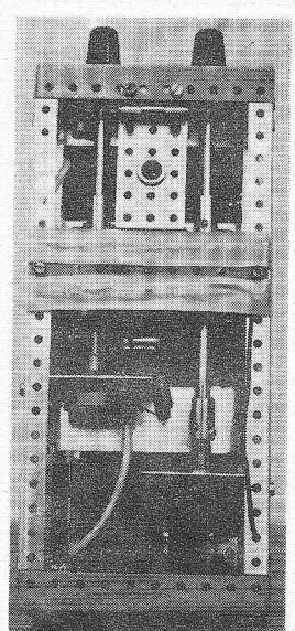
Afb. 5. Onderaanzicht MEV-101.
