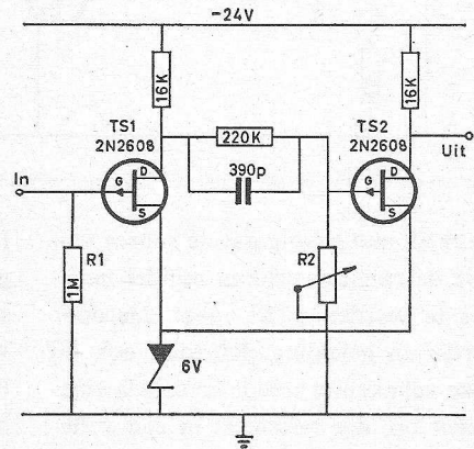
Fig. 5. Schmitt-trigger. Spanningszwaai aan de uitgang — 6 ... —24 V. Schakeltijden: 200 tot 500 ns. Triggerniveau (R2 = 82 kΩ): aan: 5,4 ... 5,5 V, uit: 5,35 ... 5,45 V. Hysteresis: 2 ... 5 mV.
