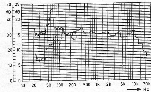
Fig. 9. Totaal geluidsdrukverloop van twee boxen, waarvan één box is omgepoold. De bovenste kromme geldt voor gelijkgepoolde boxen, de onderste voor omgepoolde. Hierbij geldt de 50 dB-schaal.
