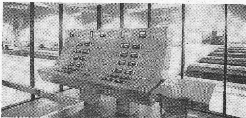
Afb. 3. Bedieningslessenaar voor niveau-regeling en terugspoeling van 24 snelfilters.
