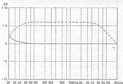
Fig. 18. Frequentie-karakteristiek MEV-101 met andere dumptrafo na één jaar bedrijf. De gestippelde lijn stelt de vermogenskarakteristiek voor (+ 6 dB = 8,7 watt)
