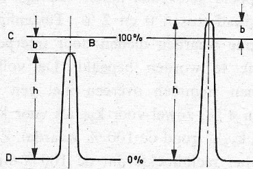
Fig. 23. Bepaling van de k_{2T/B} -factor
