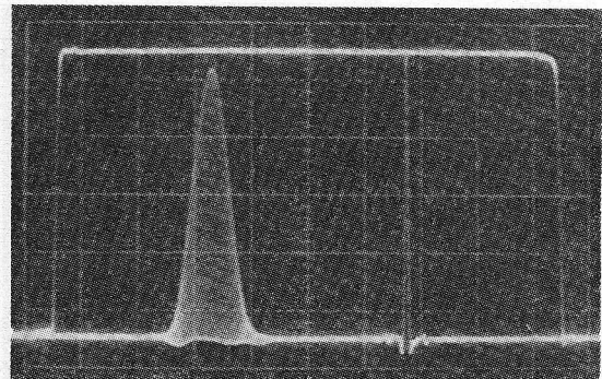
Fig. 33. Hetzelfde signaal aan de uitgang van een transmissiesysteem. De 2T-impuls vertoont de typische symmetrische overoscillatie bij grote modulatiegraden. De amplitude van de 20T-impuls is gedaald t.o.v. het kanteelsignaal (niet-lineaire vervorming)
