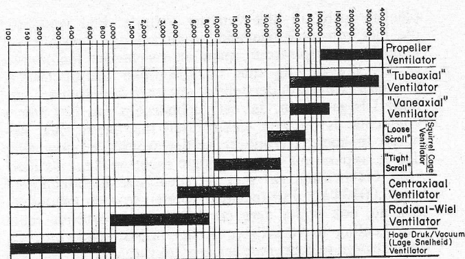
Fig. 5. Specifieke snelheid van diverse typen ventilatoren
