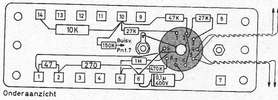
Fig. 11. Bedradingsvoorbeeld voor de 6AN8
