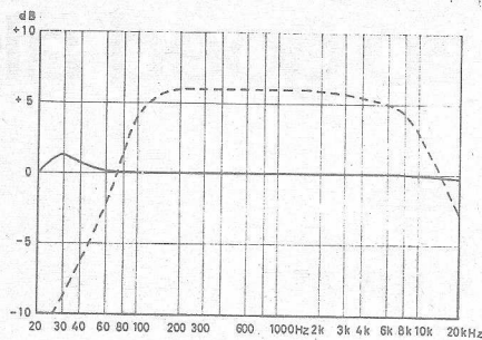
Fig. 16. Frequentie-karakteristiek MEV-101 met dumptrafo. De gestippelde lijn stelt de vermogenskarakteristiek voor (+ 6 dB = 10,08 watt).
