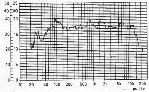
Fig. 5. Totaal geluidsdrukverloop van beide boxen. De microfoon staat op twee meter afstand in de as van de linker luidspreker. Hierbij geldt de 50 dB-schaal
