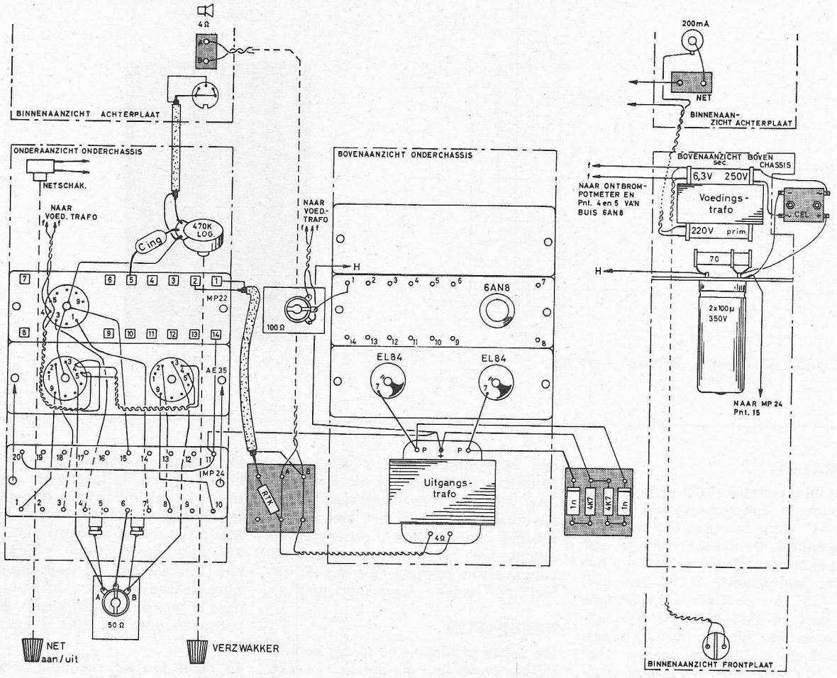
Fig. 14. Totaal bedradingschema.
