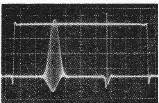
Fig. 36. Links: te hoge versterking van het HF-gebied t.o.v. de lage frequenties. De 20T-impuls vertoont ook niet-lineaire vervorming ( d_1 \neq d_2 ). De 2T-impuls is ook te groot. Rechts: de overeenstemmende frequentiecarakteristiek. Frequentiemerktekens: 500 kHz
