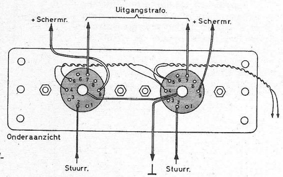
Fig. 12. Bedradingsvoorbeeld met onderdelen voor de eindtrap.
