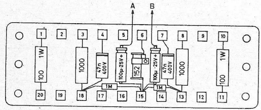
Fig. 12. Bedradingsvoorbeeld met onderdelen voor de eindtrap.
