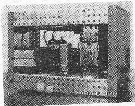
Afb. 3. Zijaanzicht van de MEV-101.
