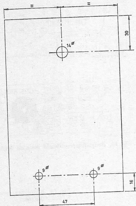
Fig. 9. Maatschets indeling van het frontpaneel.
