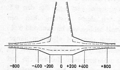
Fig. 24. Sjabloon voor het bepalen van de k_{2T} -factor. De volle lijnen stemmen overeen met een k_{2T} -factor van 4 %. De stippellijnen met 2 %. De cijfers drukken een afstand in nanoseconden uit t.o.v. de symmetrie-as van de impuls
