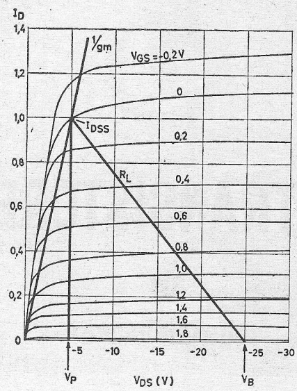
Fig. 2. Uitgangskarakteristieken met belastinglijn. V_B en V_P zijn de grenzen van het uitsturing gebied.
