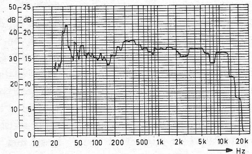
Fig. 7. Totaal geluidsdrukverloop van beide boxen. De microfoon staat op een afstand van 3 meter in het midden tussen de boxen. Hierbij geldt de 50 dB-schaal
