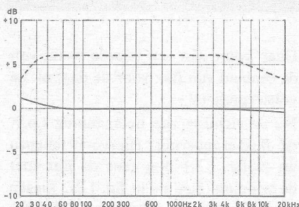
Fig. 19. Frequentie-karakteristiek MEV-101 met AMROH-trafo U60U. De gestippelde lijn stelt de vermogenskarakteristiek voor (+ 6 dB = 9,8 watt)
