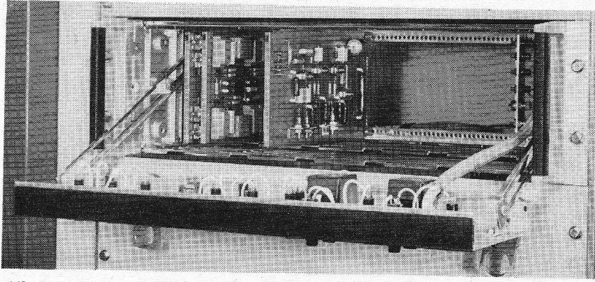
Afb. 4. Enige kaarten met gedrukte bedrading in een standaard 19-inch bak. De getoonde kaarten bevatten schakelingen voor beveiliging en vergrendeling, telschakeling en amplitude-discriminator.
